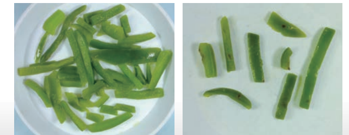
製品 Accept 排除品 Reject ピーマンの外観検査 Inspection of Pimento
